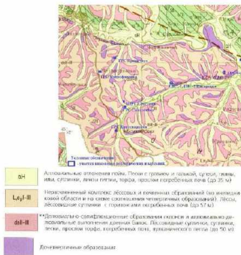
Рисунок 1 — Фрагмент схемы распространения четвертичных отложений на участках изысканий
